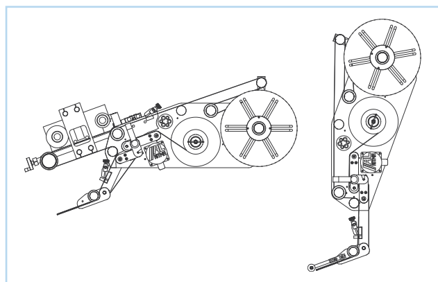
Esempi di configurazioni possibili Examples of possible configurations Esemles des configurations possibles
