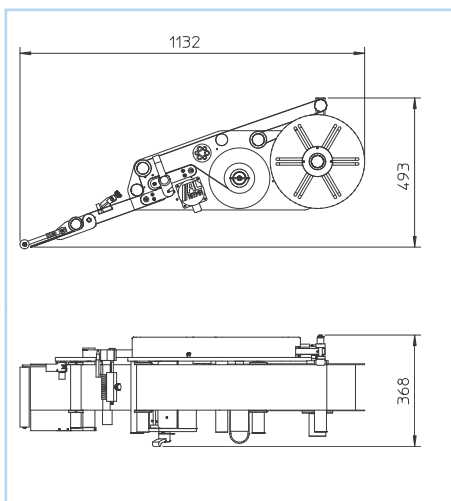
Esempi di configurazioni possibili Examples of possible configurations Esemles des configurations possibles
