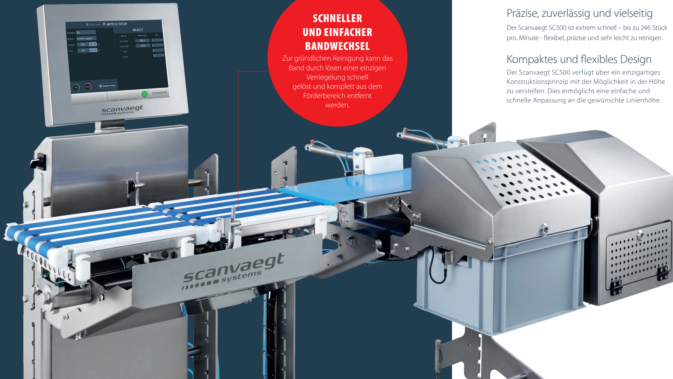
SC500 mit Metalldetektor
